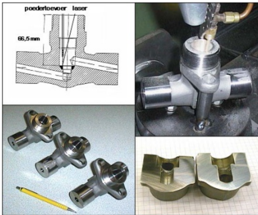
Figuur 6.8 Inwendig lasercladden van een 1/2" plugafsluiter (NedClad)
