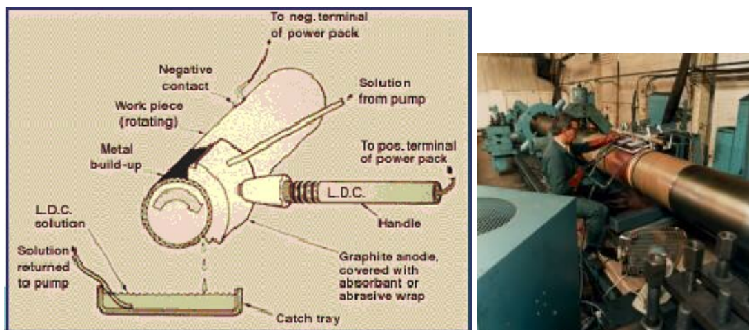
Figuur 6.17 Tampongalvaniseren, principe (bron: Maasdijk Metaal)
