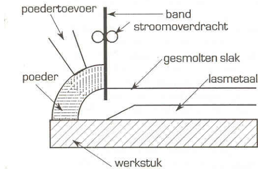
Figuur 6.1 Principeschema elektroslaglassen met band
