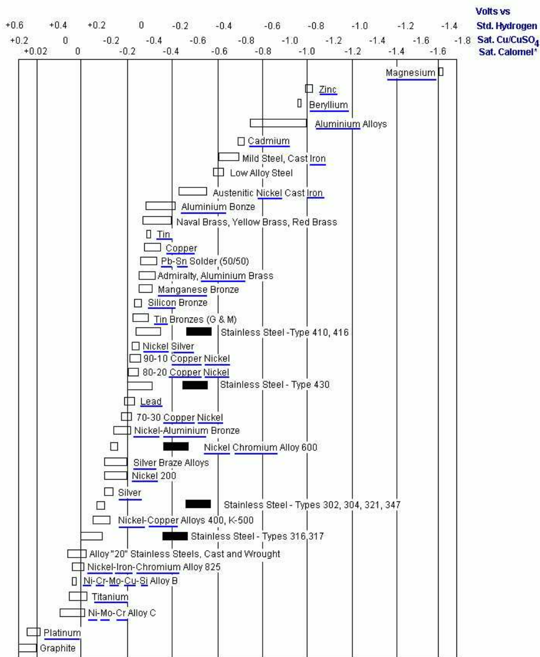
Figuur 3.7 Galvanische reeks voor metalen in zeewater. Dichte vlakken betreffen actief gedrag van het betreffende materiaal onder condities van een slechte beluchting (laag zuurstofgehalte) (ASM Handbook, vol 13 1992)
