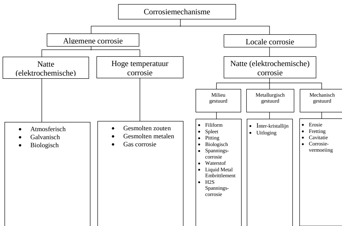
Figuur 3.6 Indeling van corrosiemechanismen
